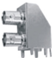
產品編號 RX.3.660.020 產品型號 BNC-K/011E/0.8
