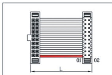
Double End-D Type
