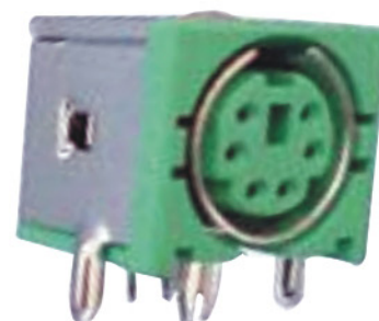
21009-4M-XXP XX:03P~08P帶魚叉+鐵圈 MINI DIN
